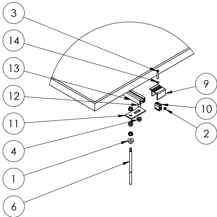
DETALHE A ESCALA 1 : 10
